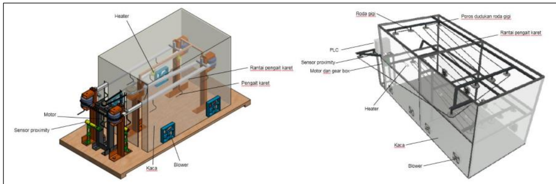
Gambar 3. 15 Desain Mesin Pengering Karet Efek Rumah Kaca Sistem Otomatis Menggunakan Programmable Logic Control (PLC).
