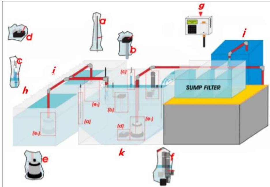
Gambar 3. 13 Desain mesin kontrol kualitas kadar air laut otomatis untuk budidaya ikan berbasis web monitoring
